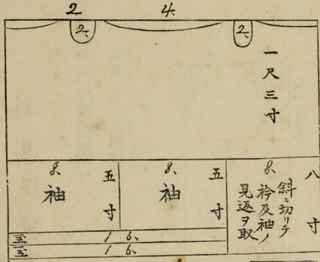
裁合綜合圖 巾二尺四寸長さ二尺一寸 (25) 西洋前掛 丙 裁方分解圖
