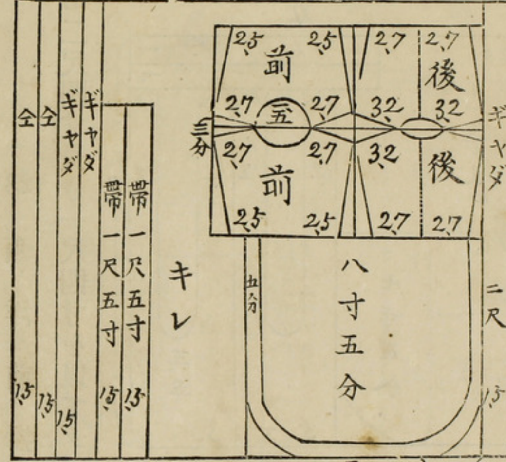
裁方綜合圖 巾二尺四寸長さ二尺にて四五歳西洋前掛裁方 (24) 西洋前掛 裁方分解圖
